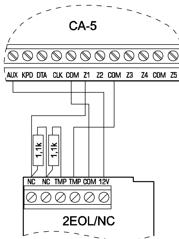
Rys. 9. Przykład podłączenia do centrali czujki typu NC w konfiguracji 2EOL (czujkę typu NO podłącza się identycznie).
