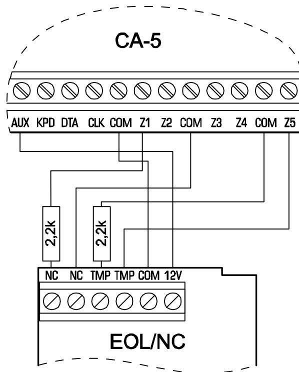
Rys. 8. Przykład podłączenia do centrali czujki typu NC w konfiguracji EOL.
